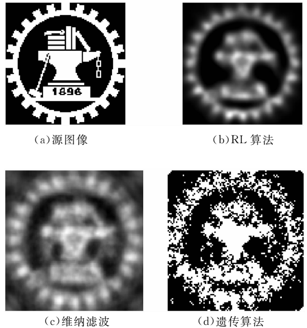
图 6 线度 10 mm 的“西安交通大学校徽”源图像及其重建图像
